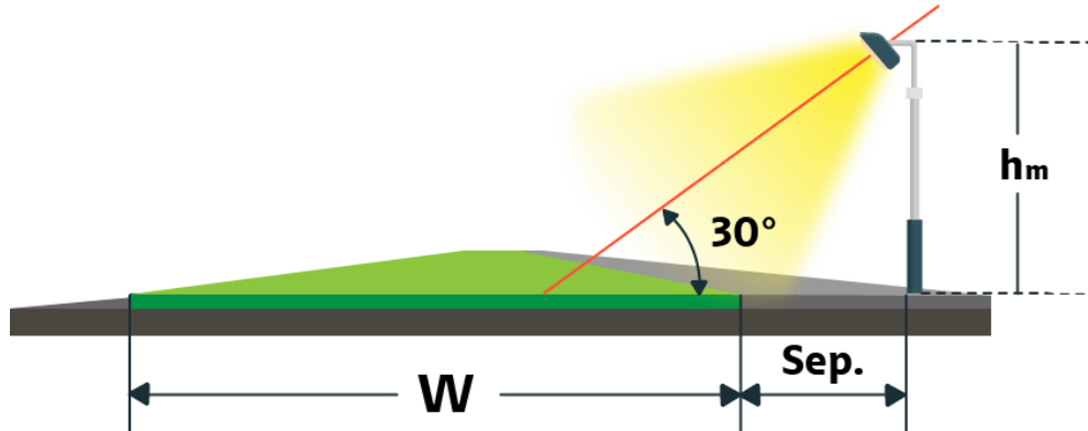
Figura 3.4.2.1. a. Diagrama que muestra el ángulo máximo de inclinación de los equipos a instalar en campos de juego exteriores sin transmisión de TV. (Fuente propia)
