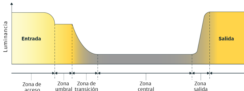
Figura 3.5.1 a. Zonas principales de un túnel. (Fuente propia)
